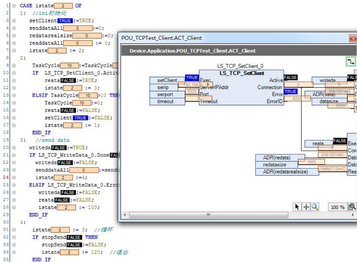
图4.72 设置客户端连接模式
