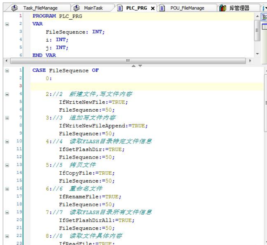
图4.8 文件操作主程序
