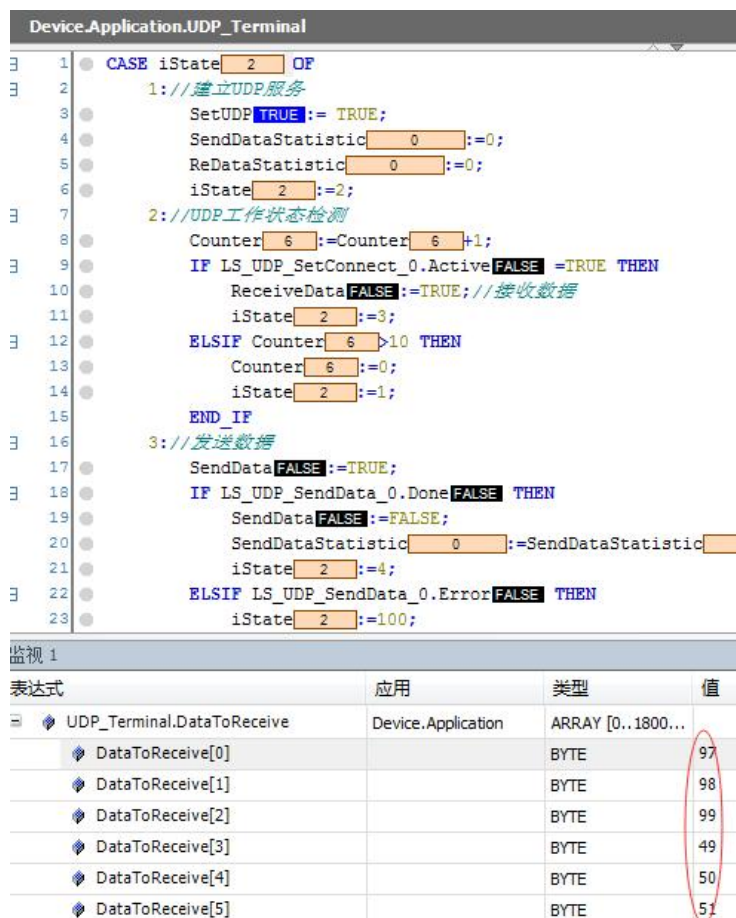
图4.79 控制器端接收来自PC端的数据
