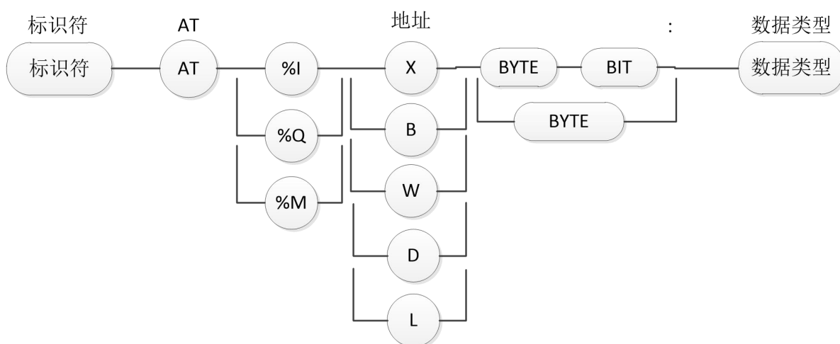
图1.2 直接变量声明的具体格式
