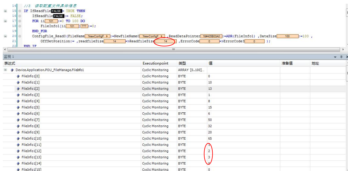
图4.36 读文件内容
