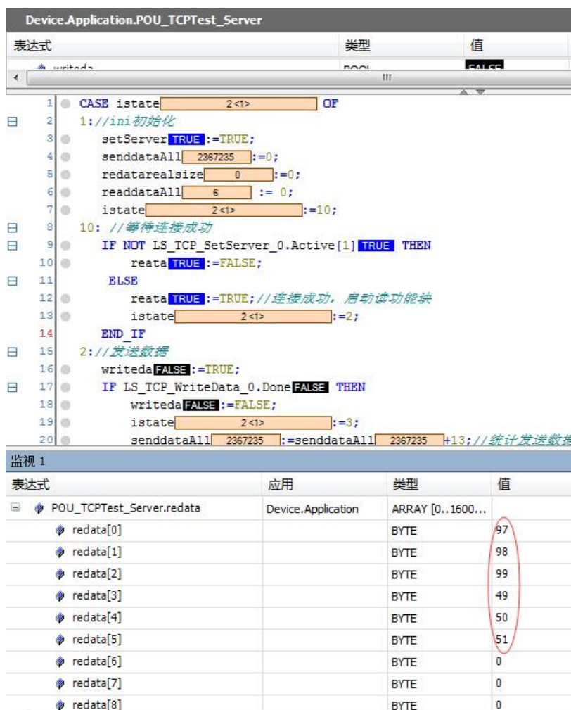
图4.70 解析数据程序
