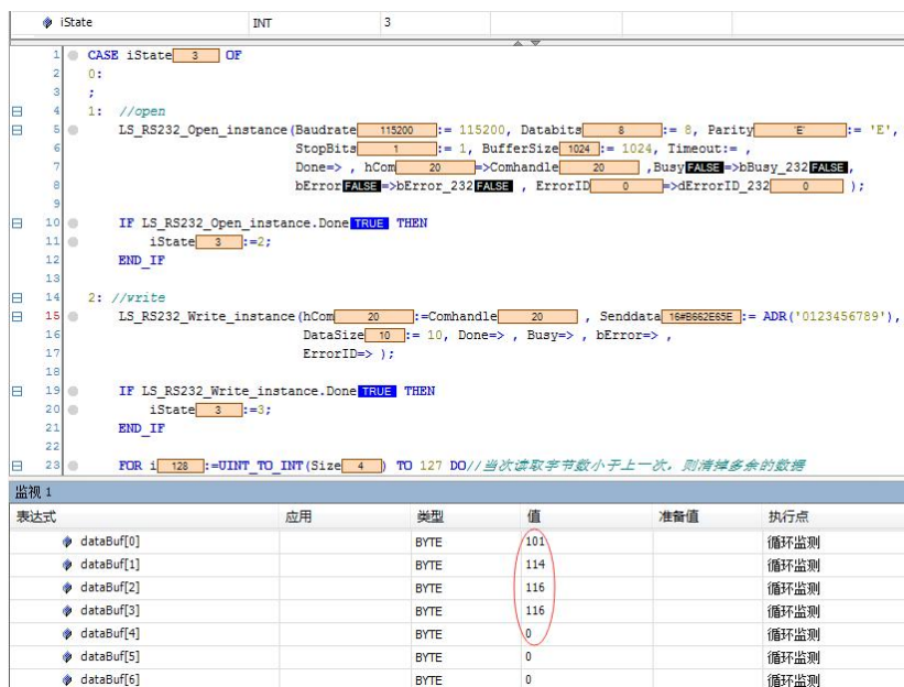
图4.63 RS232通讯控制器端接收数据
