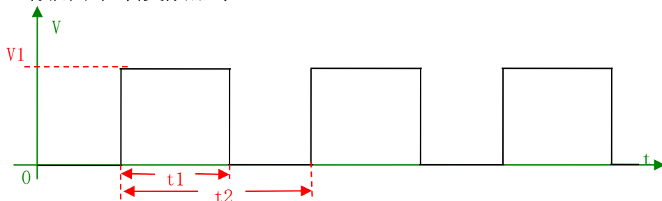
图4.1 PWM输出示意图
