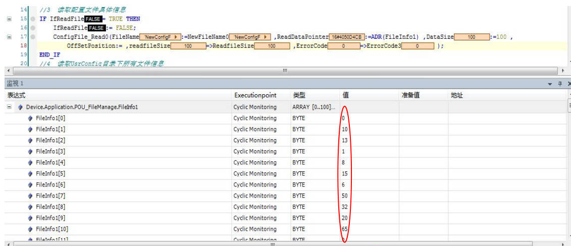
图4.34 读文件内容
