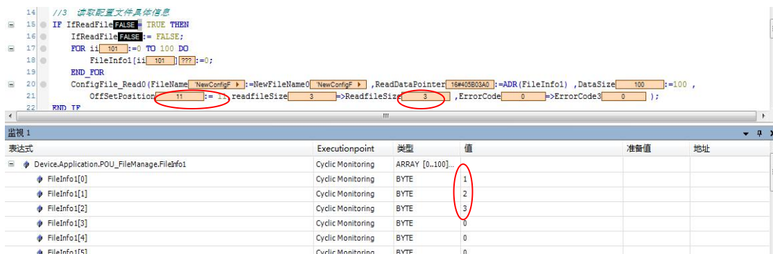
图4.37 读文件内容
