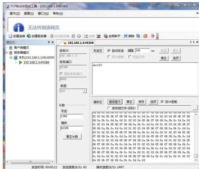
图4.73 启动服务器
