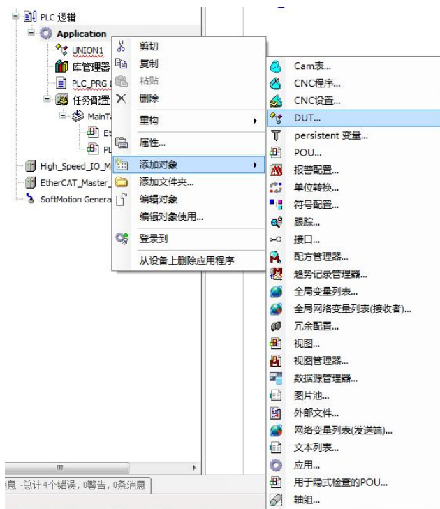
图1.4 添加结构体
