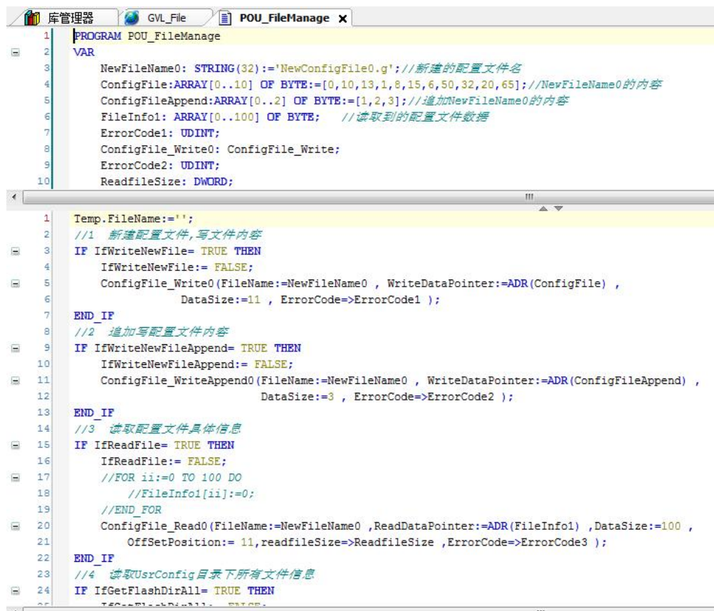
图4.29 UsrConfig文件操作模块主体
